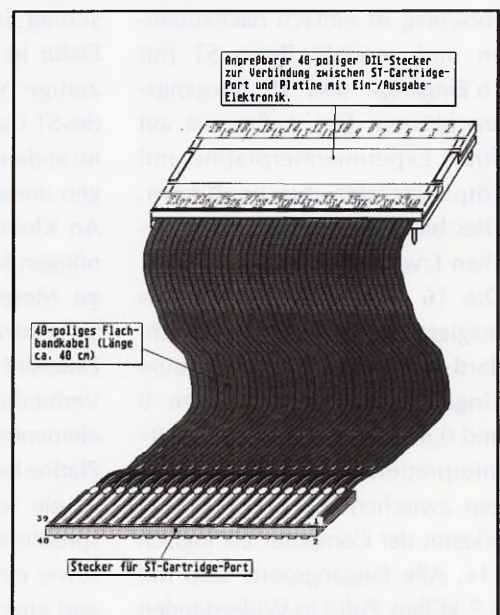
Bild 3. Die Verbindung zwischen ST-Cartridge-Port und Platine
