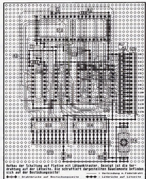
Bild 2. Der Verdrahtungsplan für die Platine
