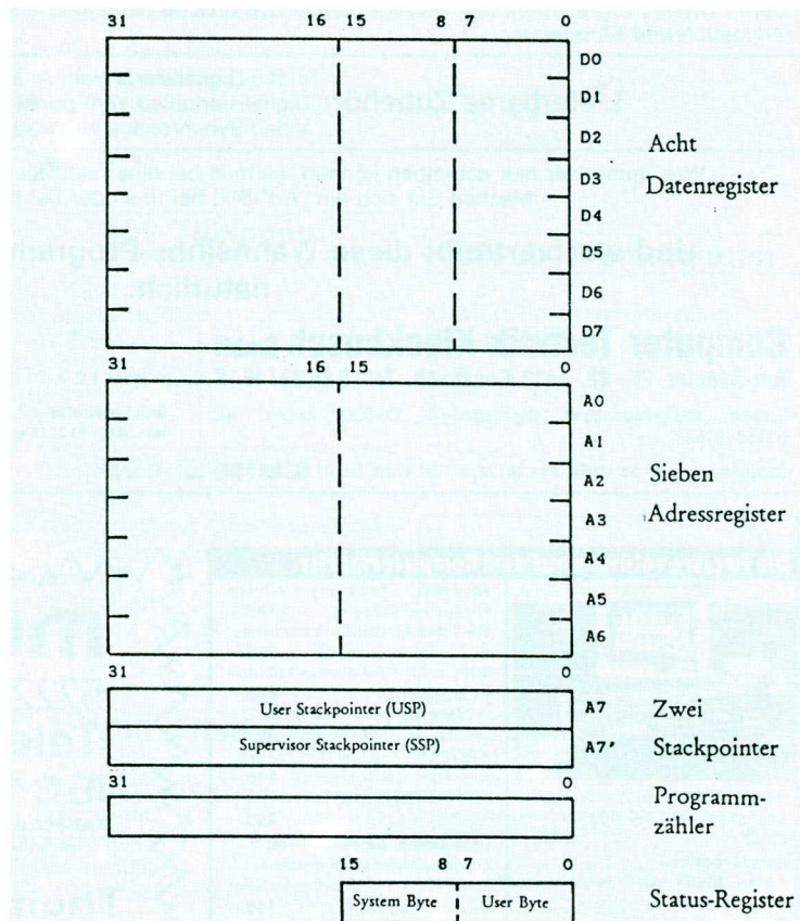
Bild 1: Die Register des 68000
