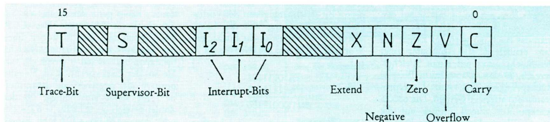
Bild 2: Das Statusregister des 68000
