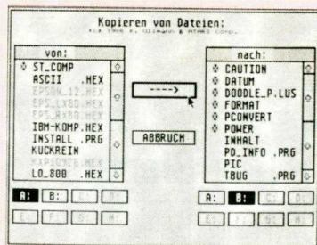
MMCOPY.ACL (PD13)
