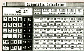
Taschenrechner (PD12)
