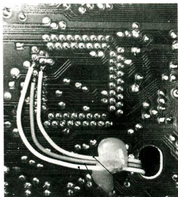
Bild 6: MMU CASH Pin 22 CASL Pin 21 Pin 18 RAS
