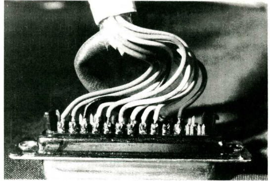
Bild 3: Cannon-Stecker
