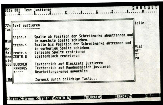
Bild 9: Beispiel eines Help-Fensters
