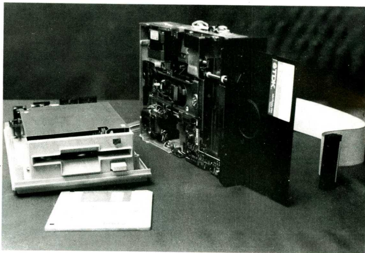
Bild 1: ATARI Floppy mit einem 5 1/4-Zoll Laufwerk gekoppelt
