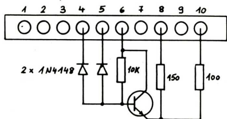
Schaltung zur Erzeugung des Composite Synchron-Signales. (Für den 520 ST)
