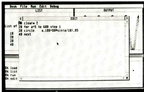
Bild 2: Das Edit-Fenster
