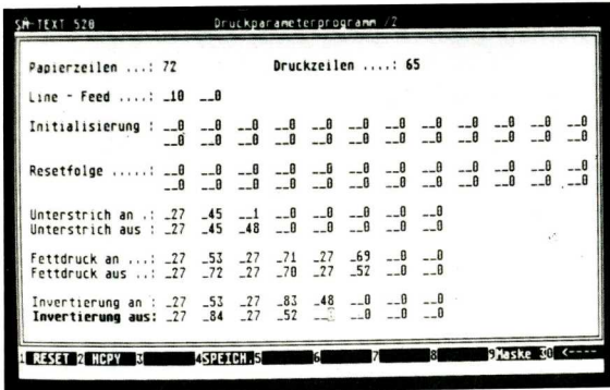
Bild 7: Druckeranpassung
