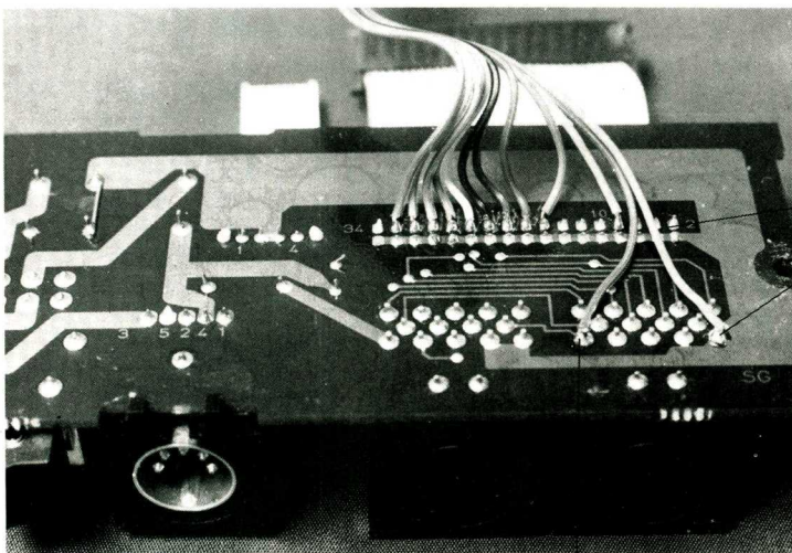
Bild 2: Anschlußplatine der ATARI Floppy von unten gesehen
