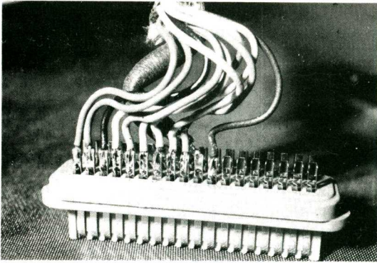
Bild 2: Amphenol-Stecker
