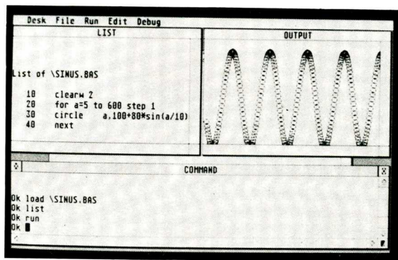
Bild 1: Die 4 Fenster des BASIC
