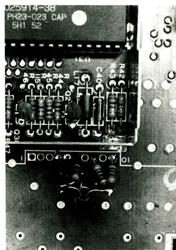
Aufbau der nebenstehenden Schaltung
