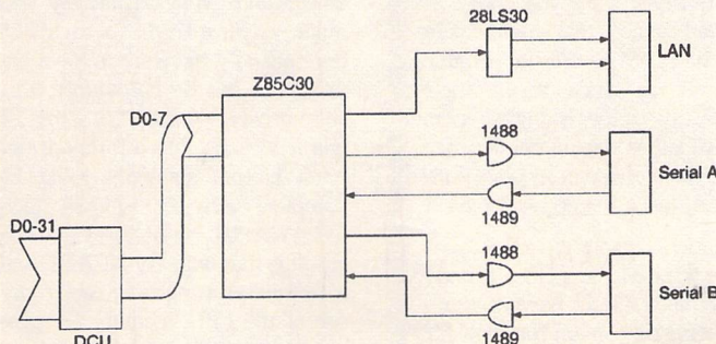
Figure 7 LAN
